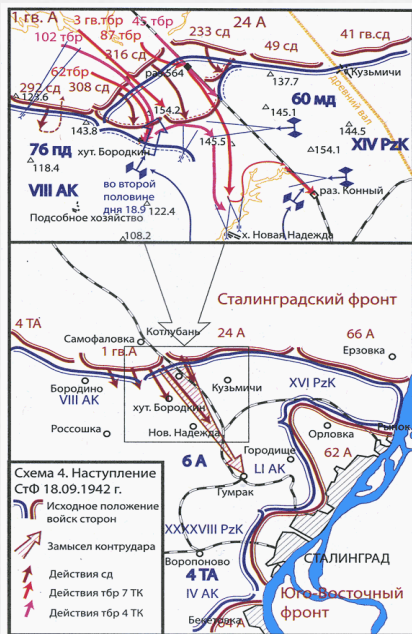
Схема боевых действий 18-20 сентября 1942 года, советский контрудар
